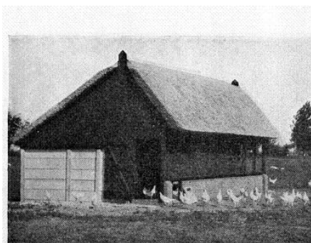
Zadeldakmodel met schuifglas (type B)
